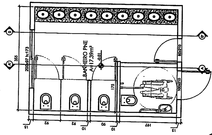
PLANTA BAIXA ESC.: 1/75
